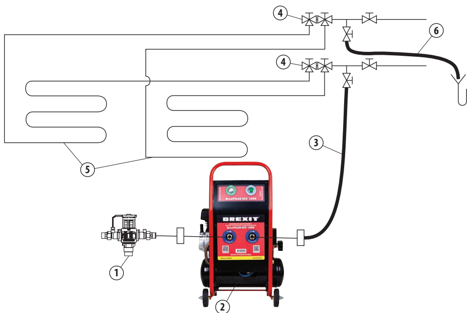
Схема подключения для промывки систем напольного отопления
